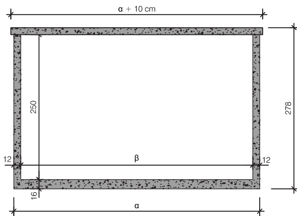
Langdoorsnede
