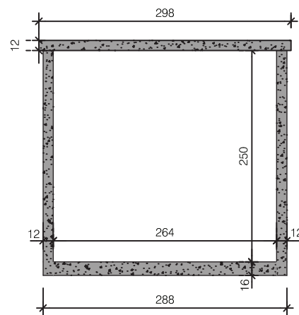
Dwarsdoorsnede
